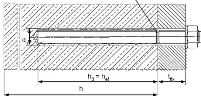
Маркировка глубины установки
